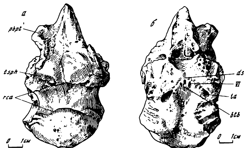
Рис. 10. Мозговая коробка анкилозаврида Maleevus disparoserratus (Maleev). Экз. ПИН, N 554/2—1; Ширэгин-Гашун; верхний мел, банширээнская свита
