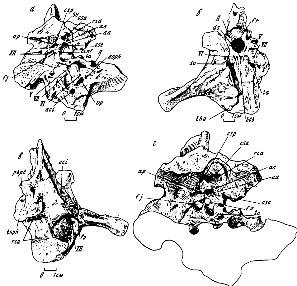
Рис. 7. Мозговая коробка анкилозаврида Talarurus plicatospineus Maleev. Экз. ПИН, N 3780/1; Байшин-Цав; верхний мел, банширэнская свита
