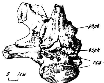
Рис. 8. Мозговая коробка анкилозаврида Pinacosaurus grangeri Gilmore (снизу). Экз. ПИН, N 4043; Бага-Тариач; верхний мел, джадохтская свита Обозначения см. на рис. 7
