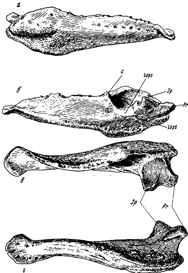
Рис. 12. Правая ветвь нижней челюсти Shamosaurus scutatus Tumanova. Экз. ПИН, N 3779/2—2; Хамрын-Ус; нижний мел, дзунбаинская свита
