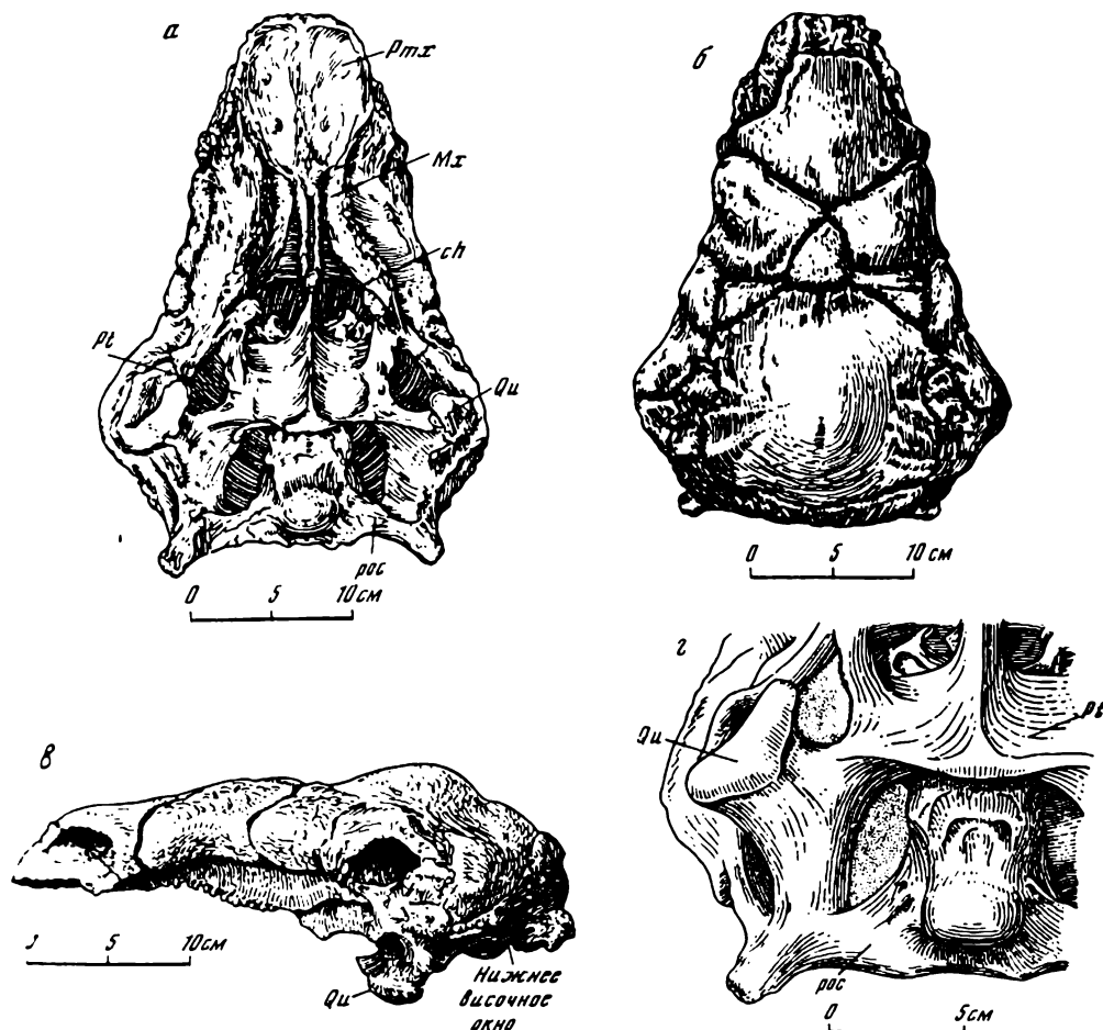
Рис. 1. Череп нодозаврида Panoplosaurus mirus Lambe. По У. Кумбсу (Coombs, 1978)
