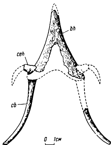
Рис. 13. Гиоидный аппарат анкилозавра Saichania chulsanensis Maryanska. По Т. Марианской (Maryanska, 1977)
