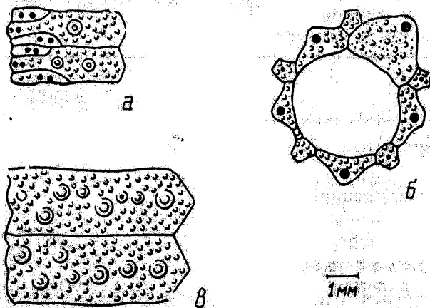
Codechinus prosorowskyi Poretzkaja, sp. nov.: а — амбулакральные (олигопоровые, диадематоидные) пластинки; б — строение апикального поля; в — интерамбулакральные пластинки (ниже амбитуса).
