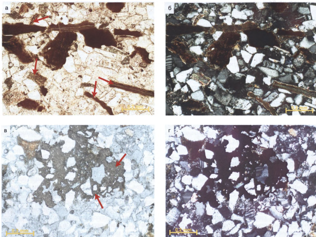
Рис. 3. Песчаники мелкозернистые алевритистые полевошпат-кварцевые с глинистым пленочно-поровым цементом: микрофотографии песчаника из нижней части тигянской свиты в параллельных (а) и скрещенных (б) николях, стрелки указывают на пластинки железистых гидрослюдов; микрофотографии песчаника из средней части тигянской свиты в отраженном свете (в) и скрещенных николях (г), стрелки указывают на агрегат тонких глобулярных стяжений пирита
