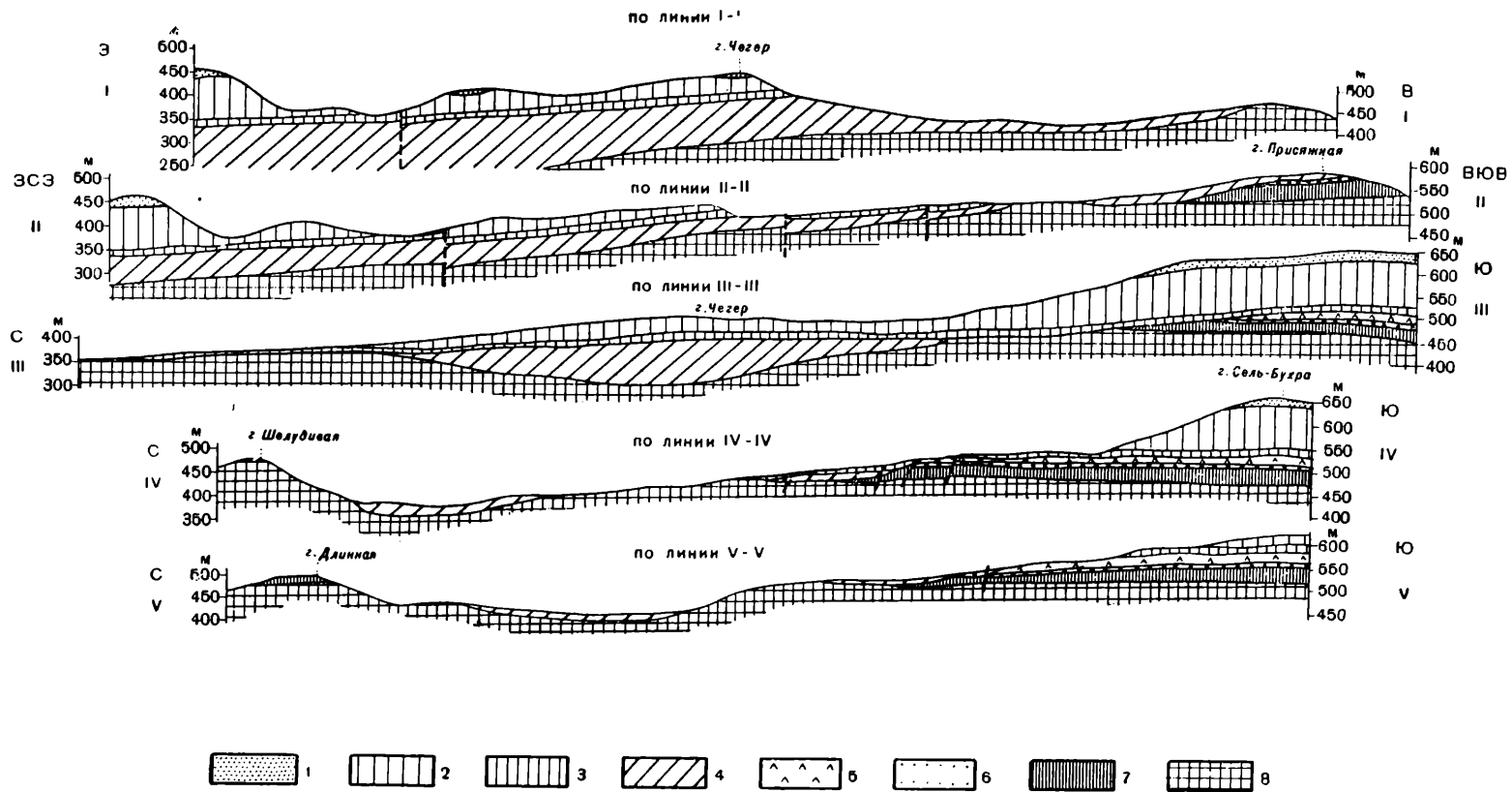
Рис. 2. Схематические геологические разрезы окрестностей с. Прохладного. Условные обозначения 1—8 те же, что на рис. 1
