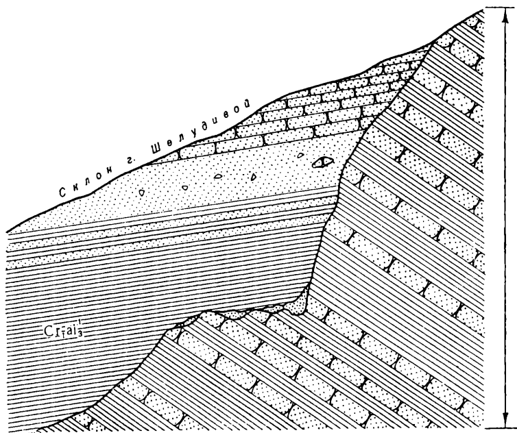
Рис. 3. Контакт прилегания глин и песчаников зоны Hysterocheras orbigny (Cr 1 al 3 ) к аргиллитам и алевролитам таврической серии (J 1 ) на южном склоне горы Шелудивой
