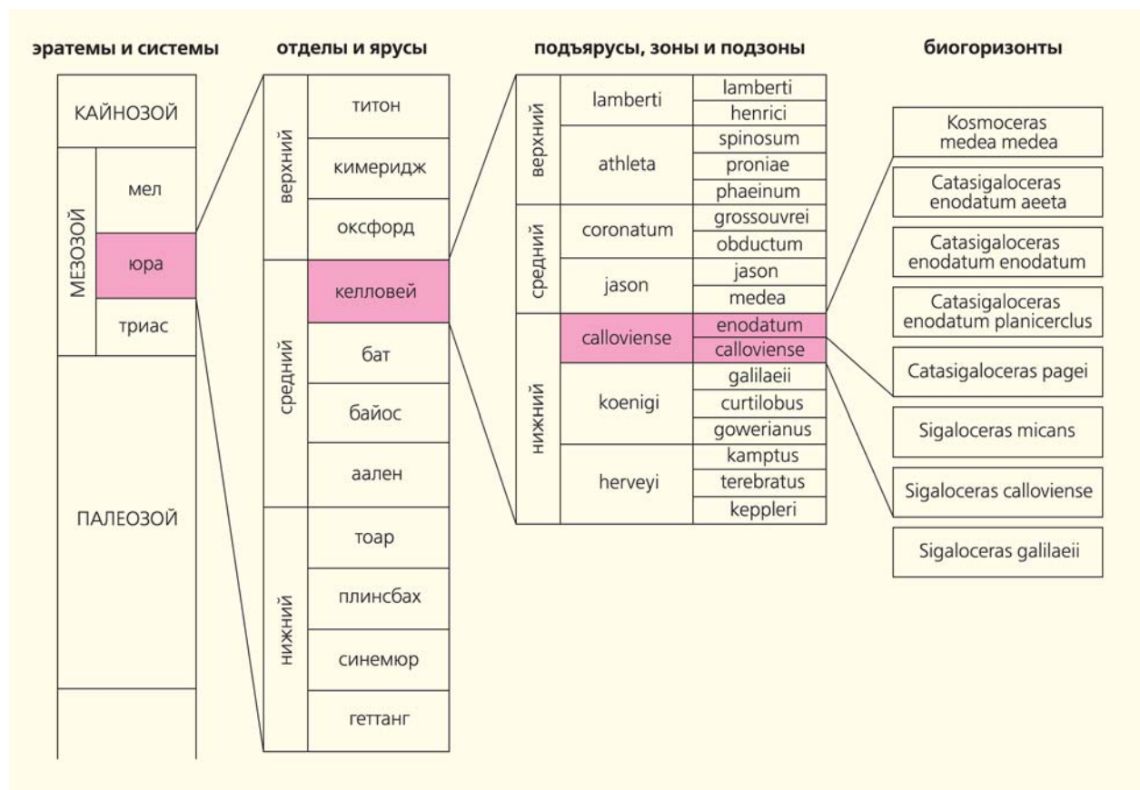
Рис.1. Фрагмент геохронологической шкалы. Приведена схема детализации шкалы келловейского яруса (подъярусы, зоны, подзоны и биогоризонты) юрской системы. На основе биостратиграфического метода проводилось исследование развития во времени (филогенезов) и расселения по акваториям (миграций) аммонитов.
