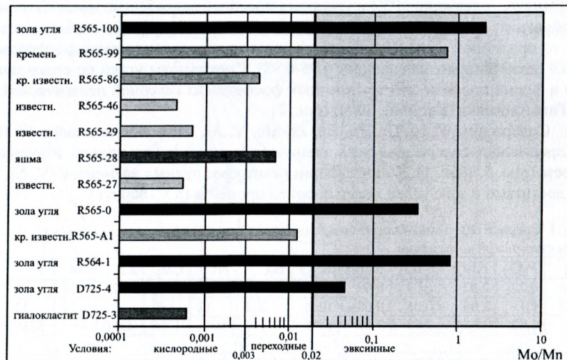
Рис. 8. Отношения Mo/Mn в породах смагаинской ассоциации. Условия осадконакопления в соответствии с коэффициентом Mo/Mn (по В.Н. Холодову, Р.И. Недумову, 1991).
