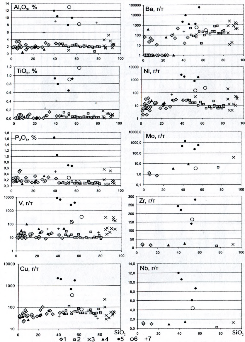
Рис. 5. Содержание некоторых элементов в породах смагинской ассоциации на диаграммах \text{SiO}_2 – элемент. 1 – розовые известняки, 2 – красные яшмы, 3 – серые кремни, 4 – серые известняки, 5 – зола углей, 6 – гиалокластиты, 7 – кремни и известняки с примесью гиалокластиты.
