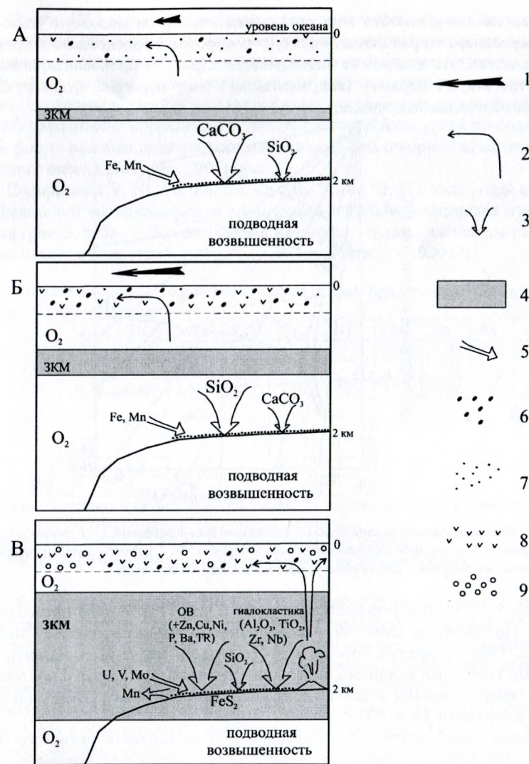
Рис. 6. Модель осадконакопления при формировании смагинской ассоциации. А – отложение карбонатных илов, Б – отложение кремнистых илов, В – отложение сапропелевых илов и гиадокластиков. 1 – сила ветра; 2 – интенсивность апвеллинга; 3 – поступление в осадки кремнезема, карбоната, гиадокластиков, различных хим. элементов; 4 – зона кислородного минимума и ее интенсивность; 5 – обогащение и обеднение осадка гидрогенными элементами; 6 – радиолярии; 7 – известковый планктон; 8 – бесскелетный фитопланктон; 9 – цианобактерии.
