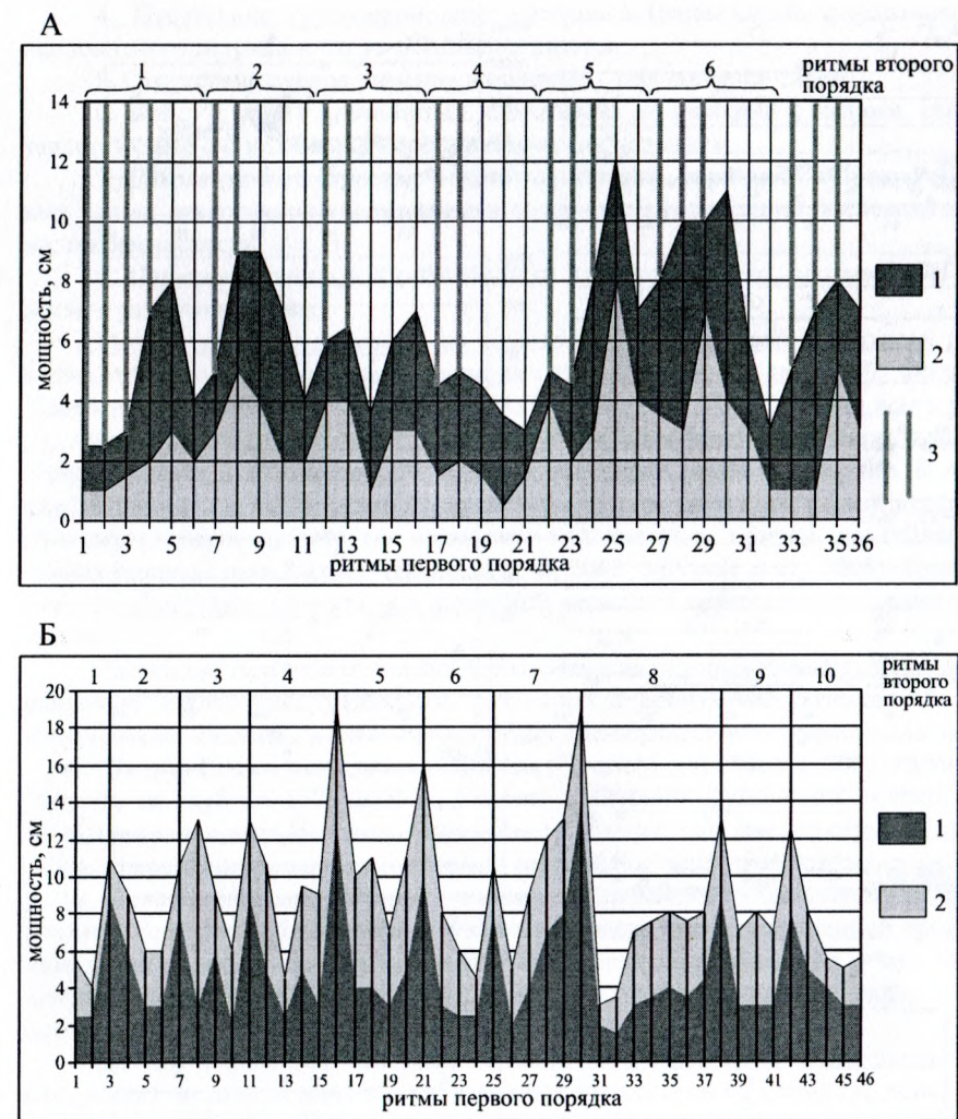
Рис. 4. Ритмограммы разреза 565. А – пакки VII-VIII, Б – пачка I. 1 – яшмы, 2 – известняки и кремнистые известняки, 3 – ритмы с повышенной кремнистостью известняков в пачках VII-VIII.
