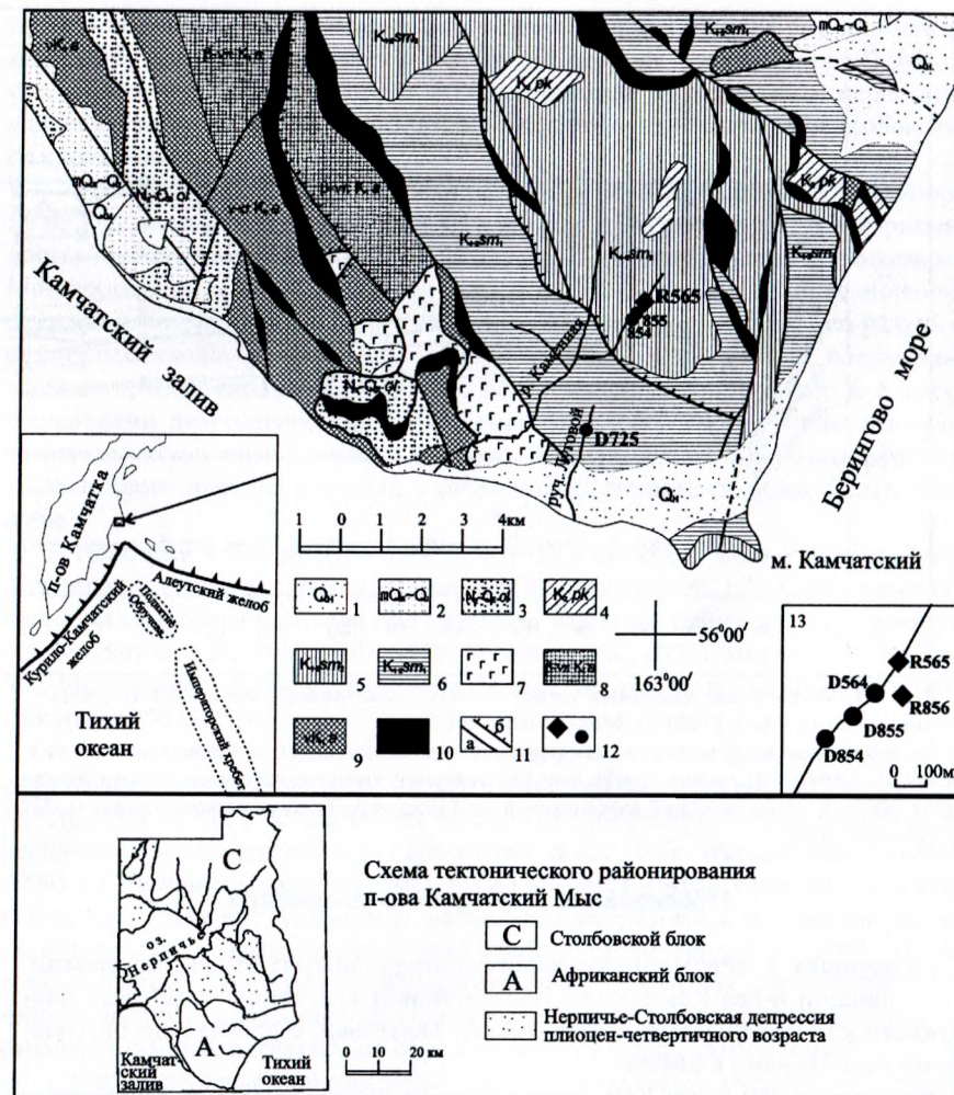
Рис. 1. Геологическая схема района исследований (по М.Е. Бояриновой, 2007) и места расположения детально изученных разрезов. 1 – рыхлые голоценовые отложения различного генезиса; 2 – эоцено-раннепалеоценовые морские отложения; 3 – плиоцен-эоценовые отложения ольховской свиты; 4 – турон-кампанские терригенные отложения пикежской свиты; 5-6 – альб-сеноманские отложения смагинской свиты (5 – нижней подсвиты, 6 – верхней подсвиты, в составе которой наблюдаются пакки или олистолиты кремнисто-карбонатного переслаивания); 7 – тектоническая пластина базальтов, отнесенная к нижней части смагинской свиты; 8, 9 – долериты (8) и габбро (9) раннемелового африканского комплекса; 10 – гипербазиты и серпентинитовый меланж; 11 – разрывные нарушения (а – недифференцированные, б – надвиги); 12 – места расположения разрезов и точек, описанных в диссертации; 13 – точки и разрезы на левом притоке р. Каменной на врезке.
