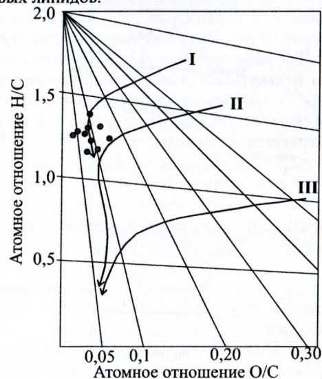
Рис. 7. Угли змагінської асоціації на діаграмі Ван-Кревелена. I – кероген морського походження; II – кероген змішанного походження; III – кероген наземного походження. Точки на графіку – положення вугілля змагінської асоціації.
