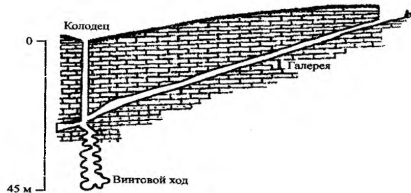
Рис. 3. Разрез колодца и подземной галереи у стен крепости Чуфут-Кале (по А.Ф. Козлову, Ю.А. Полканову, Ю.И. Шутову).
