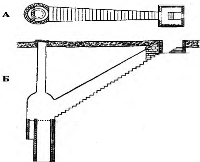
Рис. 1. План (А) и разрез (Б) колодца в районе дер. Партизаны (Керченский полуостров) (Кумурджи, 1962).
