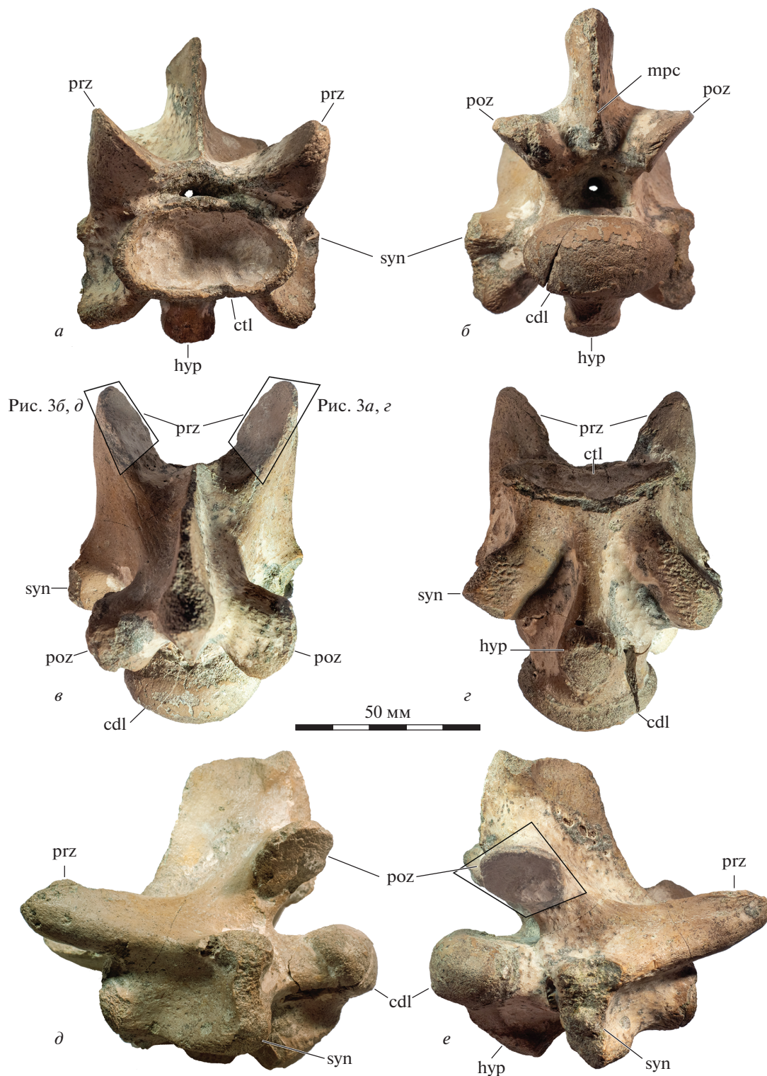
Рис. 2. Шейный позвонок Halisaurinae gen. indet., экз. ZIN PH № 29/90: а – вид спереди, б – вид сзади, в – вентральный вид, з – дорсальный вид, д, е – виды сбоку; Саратовская обл., Белое Озеро; верхний мел, нижний кампан, рыбауш-кинская свита. Полупрозрачными четырехугольниками показаны области на зигапофизах с ростовыми гребнями, изображенными крупно на рис. 3. Обозначения: cdl – задняя сочленовная поверхность позвонка, ctl – передняя сочленовная поверхность позвонка, hyp – ножка гипапофиза, mpc – задний среднесагиттальный гребень, poz – постзигапофиз, или задний сочленовный отросток позвонка, prz – презигапофиз, или передний сочленовный отросток позвонка, syn – боковой отросток позвонка.
