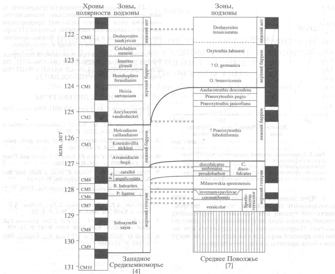
Рис. 2. Магнитохронологическая калибровка зональных шкал готерива–баррема Среднего Поволжья и Западного Средиземноморья. Условные обозначения см. рис. 1.
