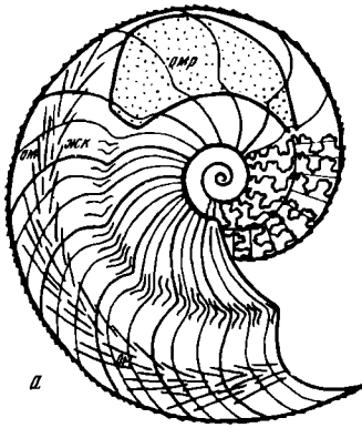
Рис. 2. Отпечатки мускулов-ретракторов у Aconeceras trautscholdi Sinz. Нижний апт, Ульяновское Поволжье. Здесь и на рис. 3: вл – вентролатеральная зона развития призматического слоя, выстилающего внутреннюю поверхность фрагмокона, дс – отпечаток дорсального мускула, жк – жилая камера, ом – отпечатки мантии, опр – отпечаток мускула-ретрактора, ф – фрагмокон
