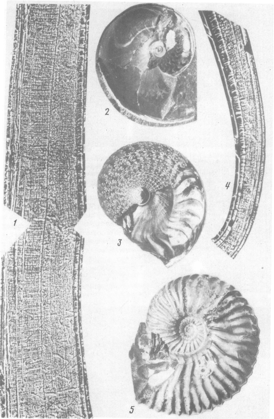
Рис. 1. 1-4 - Aconeceras trautscholdi Sinz.: 1 - микроструктура латеральной стенки задней части жилой камеры на пятом обороте (слева направо): наружный призматический, перламутровый и внутренний призматический слой, 1500 X; 2 - отпечаток мускула-ретрактора, экз. 3871/82, 5 X; 3 - отпечаток мускула-ретрактора, экз. 3871/83, 1,5 X; 4 - латеральная стенка на втором обороте (слева направо): внутренний призматический, перламутровый и наружный призматический слой, 1500 X. 5 - Deshayesites deshayesi Leum.; отпечаток мускула-ретрактора, экз. 3871/84, 1,5 X. Нижний апт, Ульяновское Поволжье
