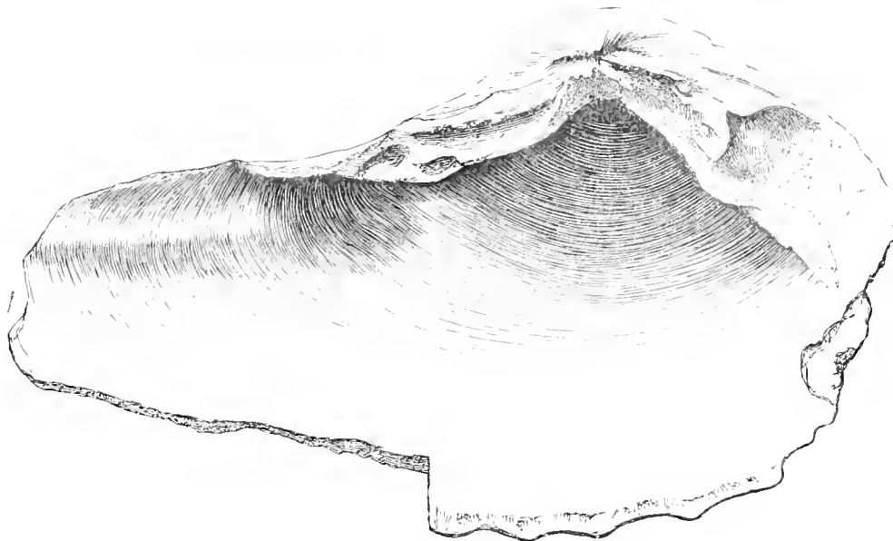
Trigonía conocardiformis , Krauss. Inner surface of valve.
