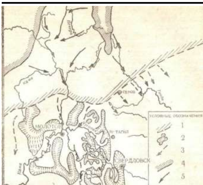
Рис. 8. Так представляют себе некоторые Мученые формирования Среднего и прилегающих к нему частей Северного Урала во время оледенений в четвертичном периоде.
