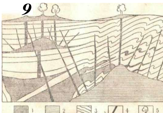
Рис. 2. На этом рисунке показаны внедрившиеся в земную кору (3) магматические очаги (1, 2) и отходящие от них жилы (4). Прорываясь на поверхность от таких очагов, расплавленная огненно-жидкая магма дает вулканы (5).
