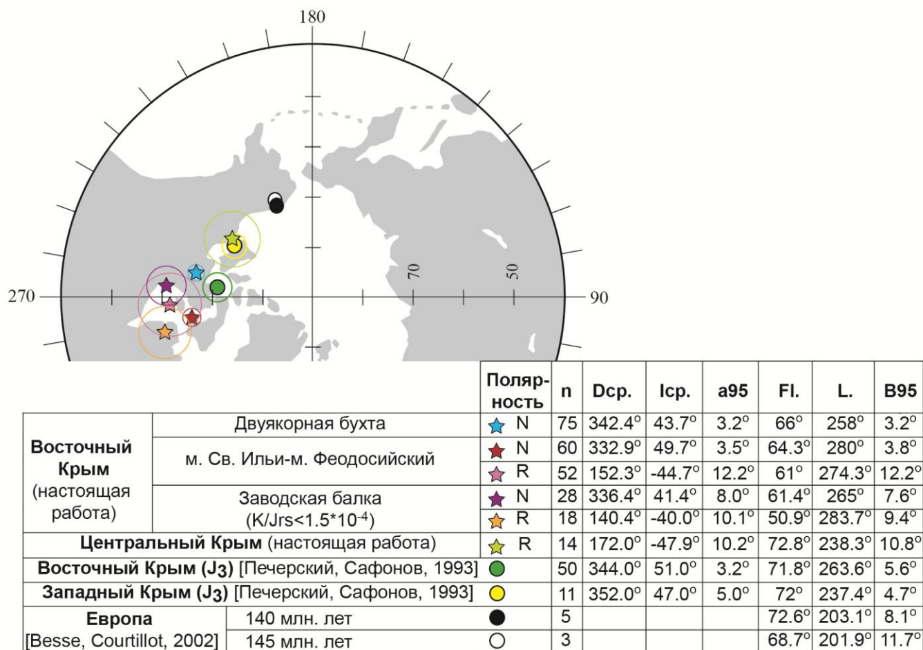
Рисунок 1 - Стереографическое изображение палеомагнитных полюсов, рассчитанных по верхнетитонским-берриасским отложениям Восточного и Центрального Крыма (настоящая работа), и верхнеюрского полюса для Восточного и Центрального Крыма [Печерский, Сафонов, 1993], стандартного полюса для Европы [Besse, Courtillot, 2002]
