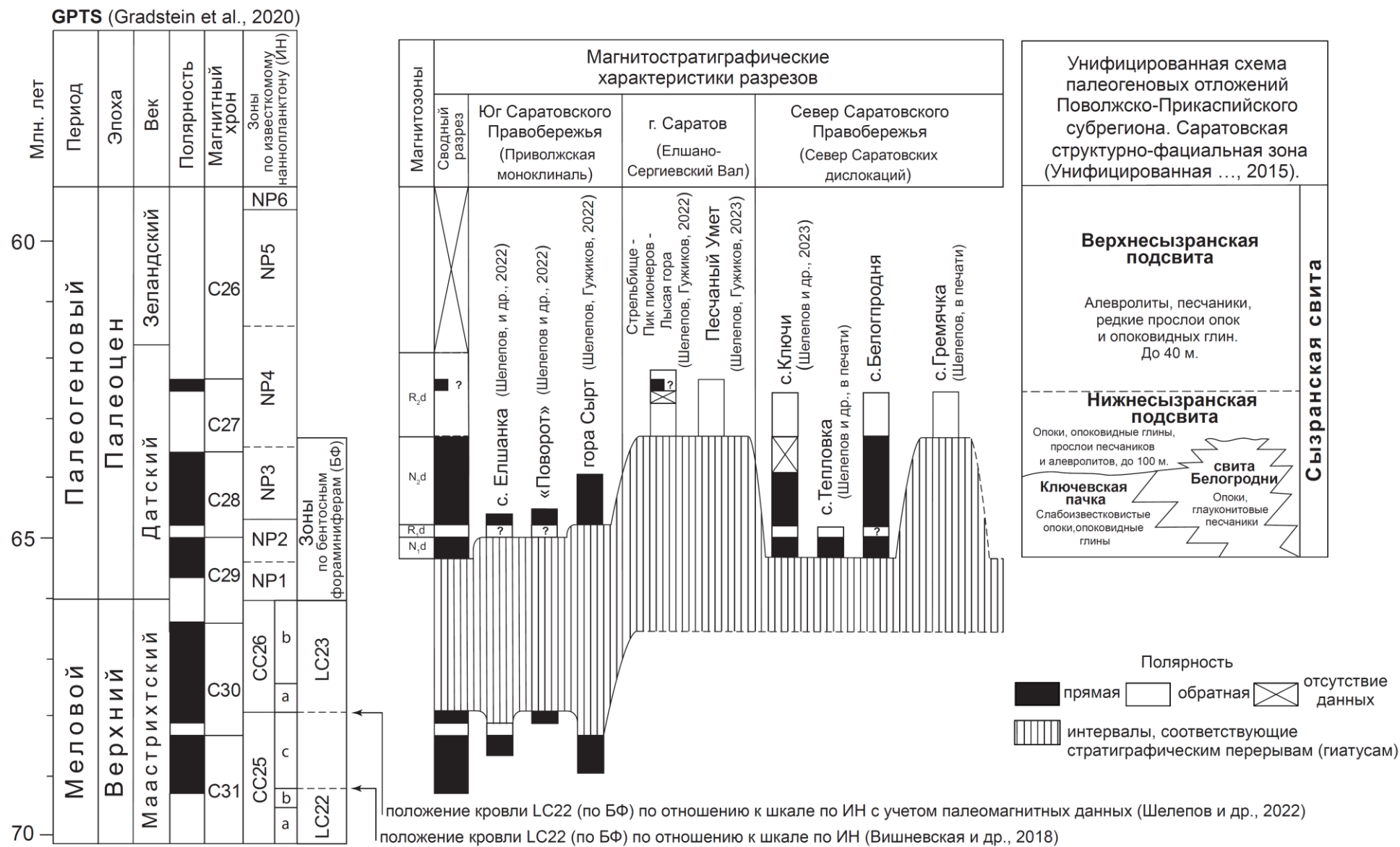
Рис. 3. Предварительная магнитостратиграфическая схема датского яруса Саратовского Правобережья.
