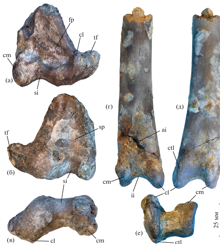
Рис. 1. Новые материалы по гесперорнисам (Aves: Hesperornithidae) из кампана местонахождения Карякино (Нижнее Поволжье, Саратовская область; верхний мел): а–в – Hesperornis rossicus Nesselov et Yarkov, 1993, фрагментарная правая бедренная кость, экз. ПИН, № 5027/8, с каудальной (а), краниальной (б) и дистальной (в) сторон; г–е – Hesperornis sp., фрагментарный правый тибиятартус, экз. ПИН, № 5027/9, с краниальной (г), каудальной (д) и дистальной (е) сторон. Обозначения: ai – apophysis internum ligament obliqui; cm – condylus medialis; cl – condylus lateralis; ctl – crista trochlearis lateralis; fp – fossa poplitea; ii – incisura intercondylaris; si – sulcus intercondylaris; sp – sulcus patellaris; tf – trochlea fibularis.
